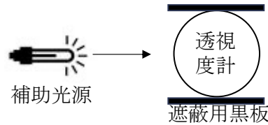
図 2: 補助光源設置例(平面図)
