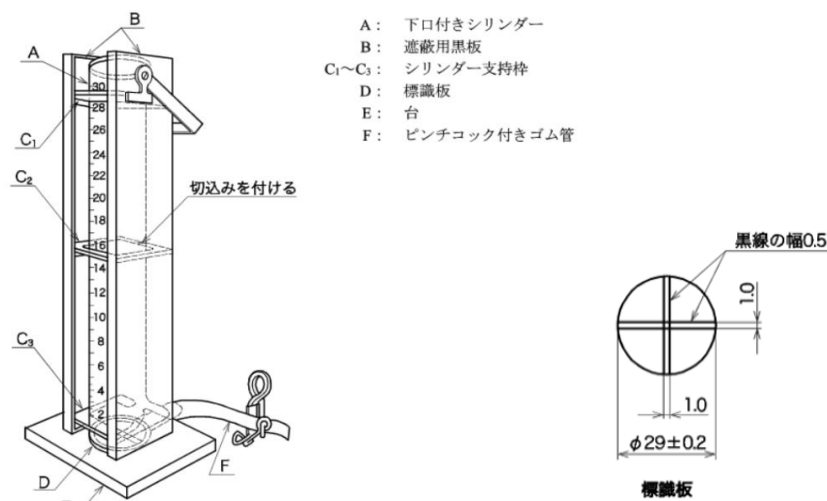
図 1：透視度計の例 (JIS K 0102:2016 図 9.1 および図 9.2 より引用転載)
